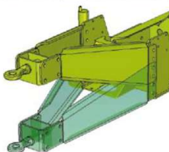
Timone ed occhione regolabile in altezza in diverse posizioni Adjustable drawbar and drawbar eye Barra de tracción y argolla regulables en altura
